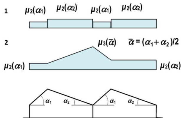
figuur 19, sneeuwbelastingvormcoëfficiënten voor daken met meer dan één overspanning volgens NEN-EN 1991-1-3, fig. 5.3
