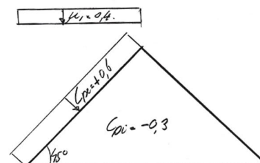
figuur 24, vormfactor uitwendige drukcoëfficiënten zadeldak 45°
